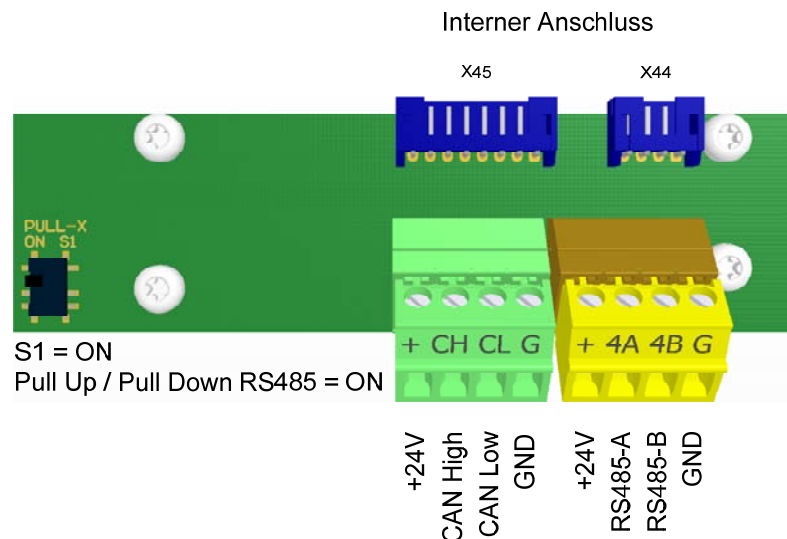
Abbildung 2: Anschlussbelegung TST RFUxFCOM
