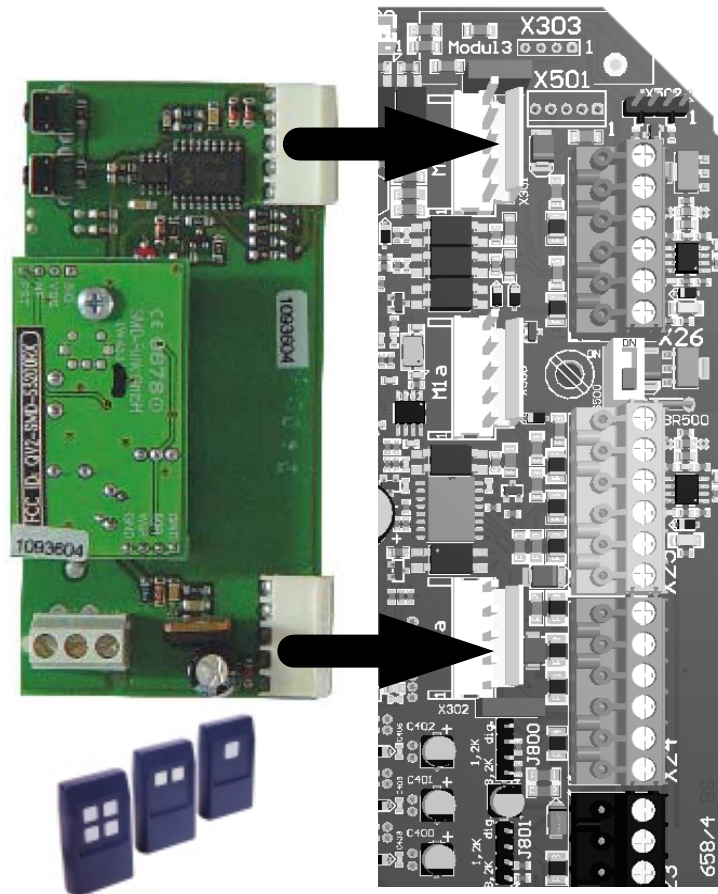
Afbeelding 35: Radio-steekontvanger
