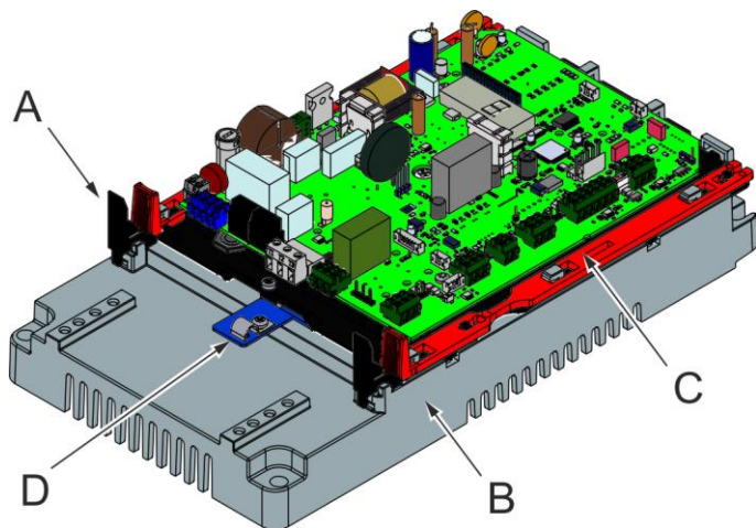
Afb. 1: Framevariant op de montageadapter
