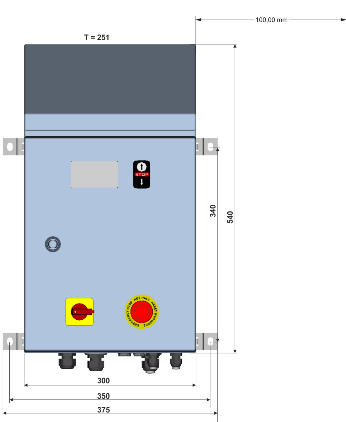
Afbeelding 14: Hygiënische behuizing (Typ: HZG)
