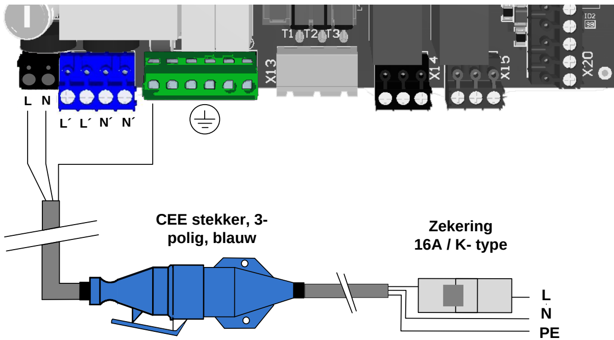
Afbeelding 16: Aansluiting netsnoer
