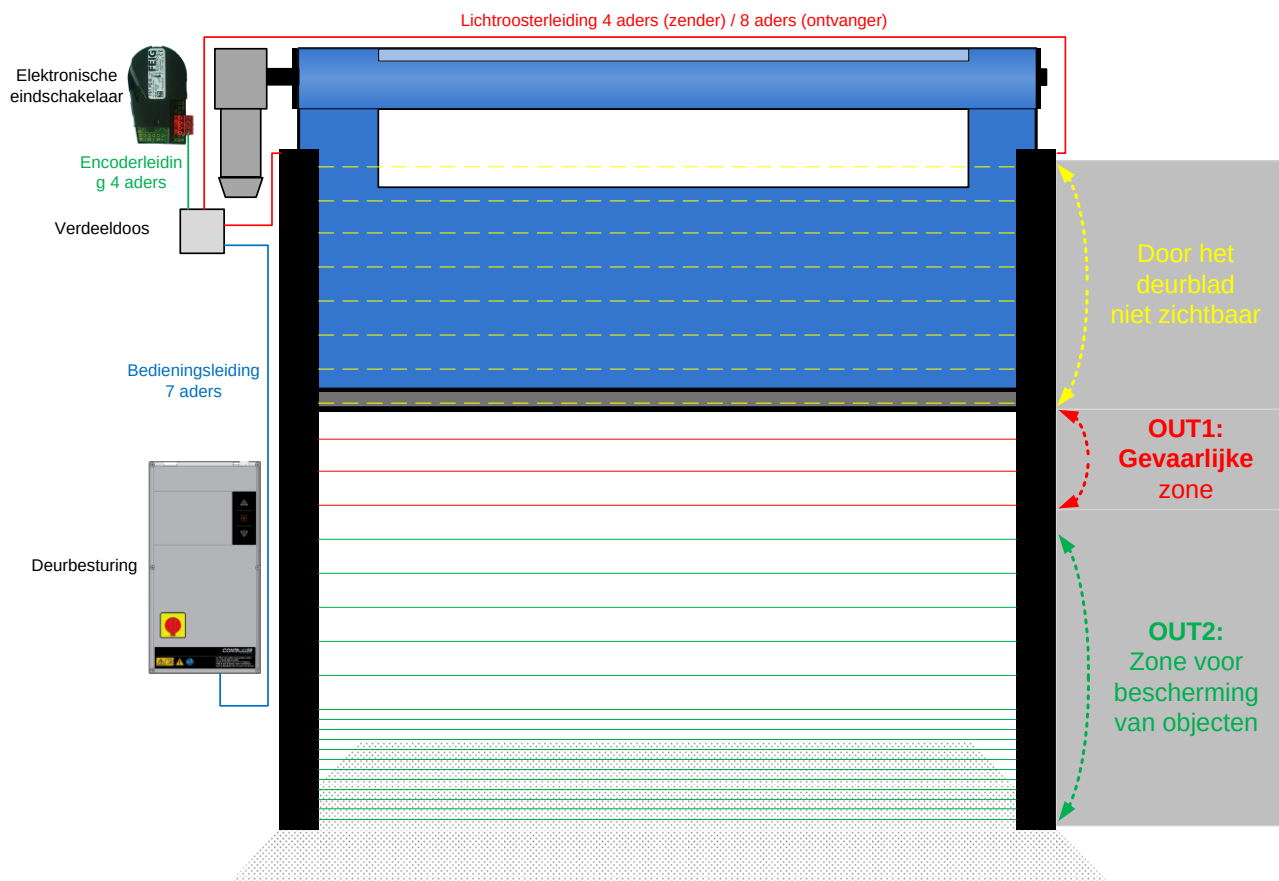
Afbeelding 24: Montage van de TST LGB
