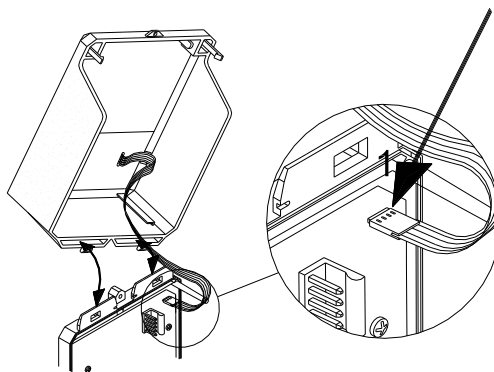
Afbeelding 6: Montagepositie van het deksel
