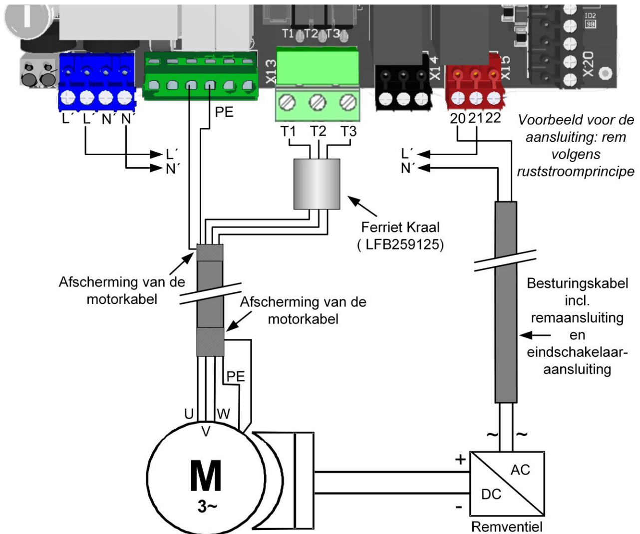
Afbeelding 18: Motoraansluiting
