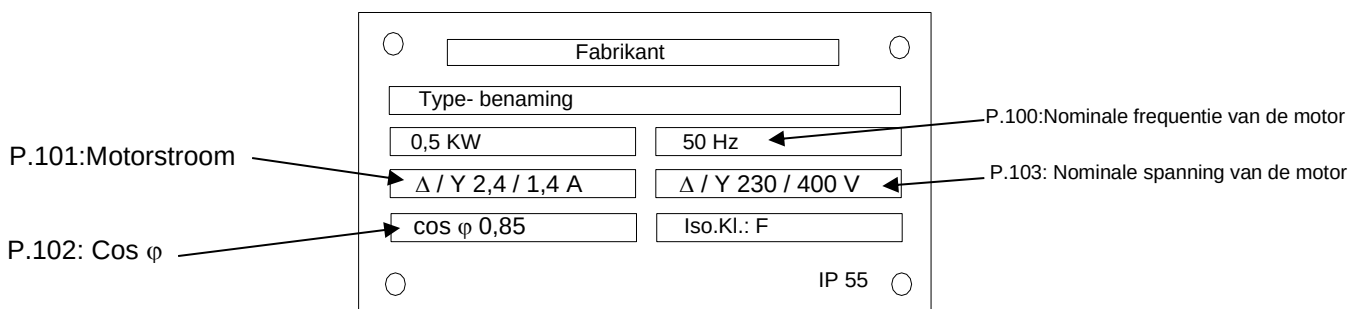
Afbeelding 45: Voorbeeld motortypeplaatje (afb. soortgelijk)
