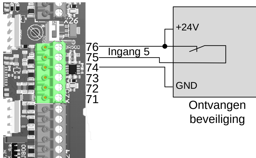
Afbeelding 30: Aansluiting foto-elektrische beveiliging
