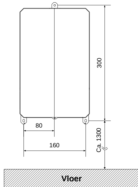
Afbeelding 5: Boorschema van kleine behuizing
