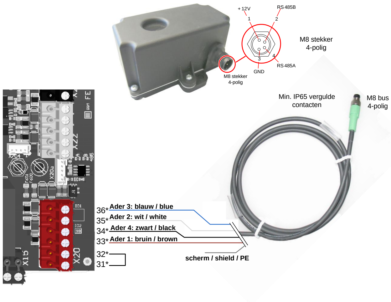
Afbeelding 27: Aansluiting van de absolute encoder TST PD
