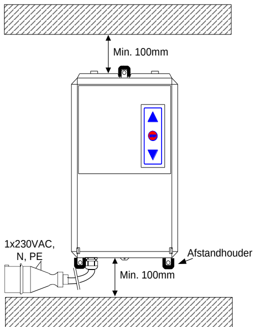
Afbeelding 4: Montage kleine behuizing
