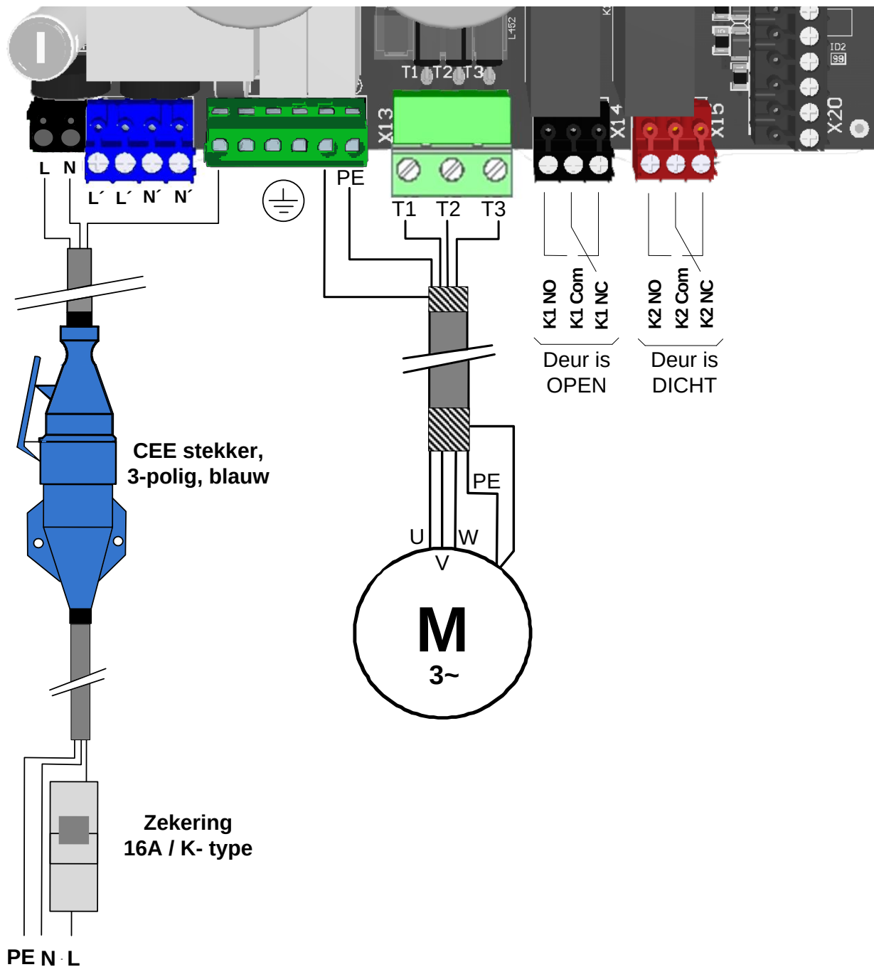
Afbeelding 33: Overzicht uitgangen
