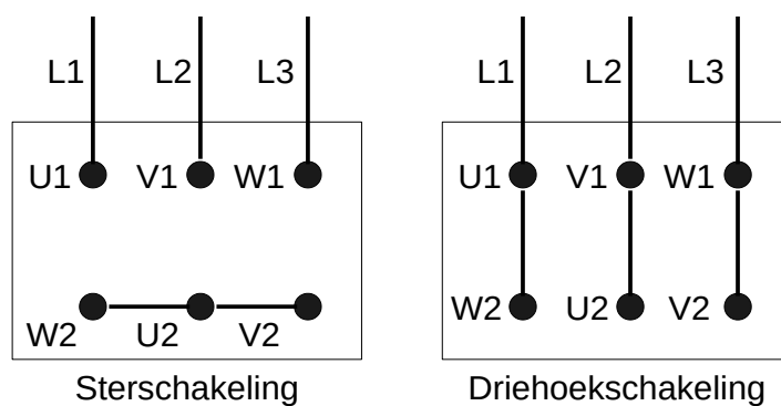
Afbeelding 46: Ster- / driehoekschakeling
