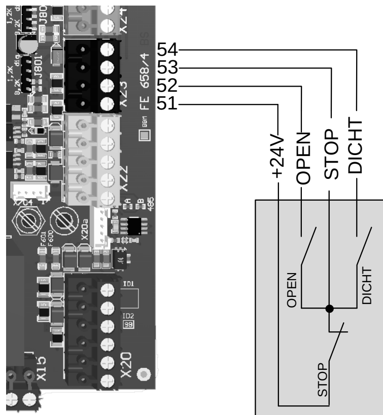
Afbeelding 31: Aansluiting van het externe commandoapparaat
