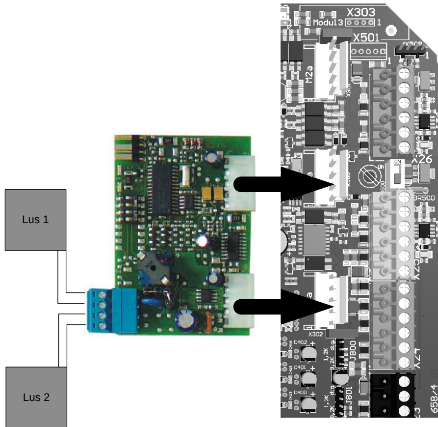
Afbeelding 36: Detectorkaart
