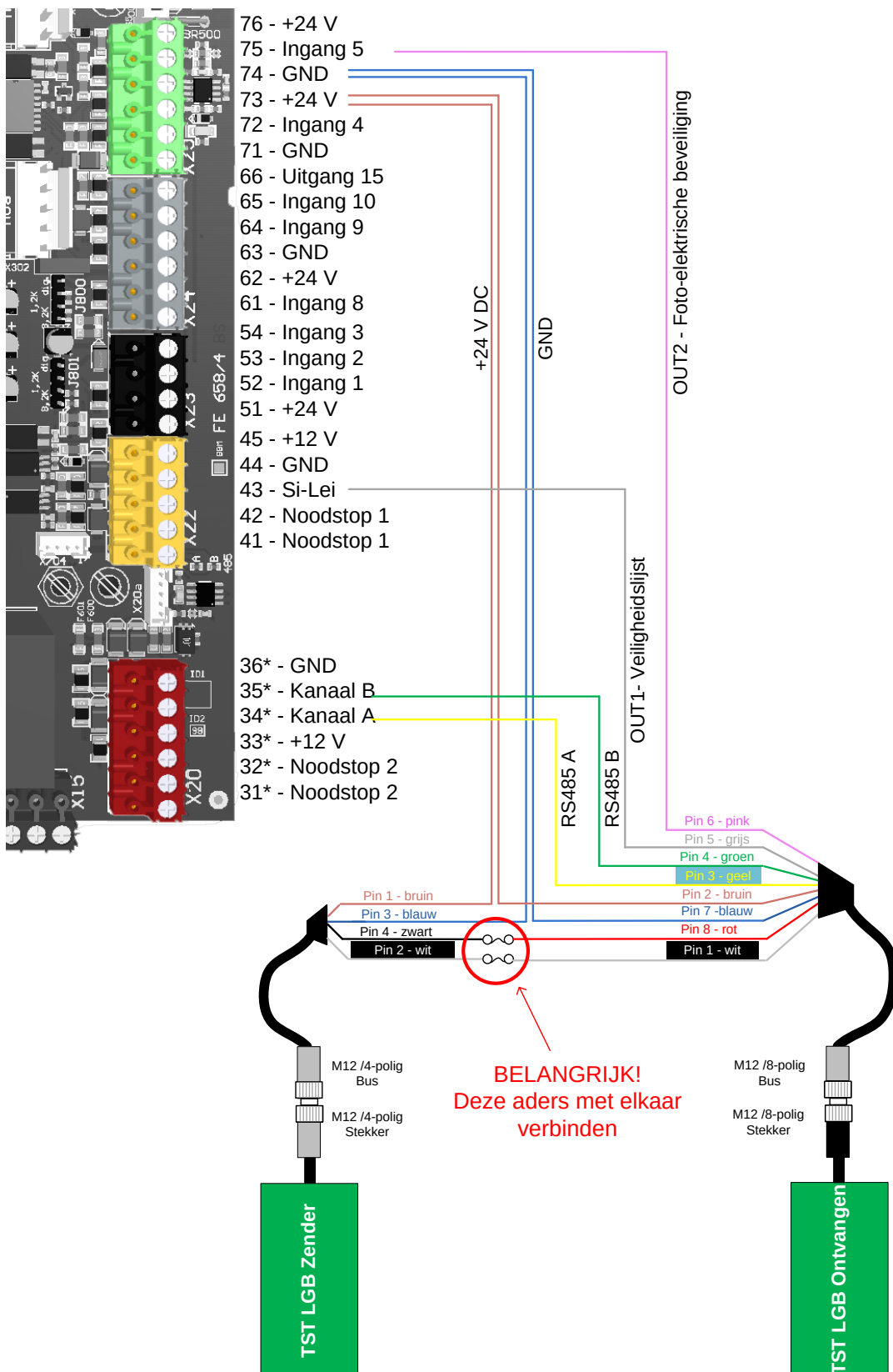
Afbeelding 25: Aansluiting TST LGB
