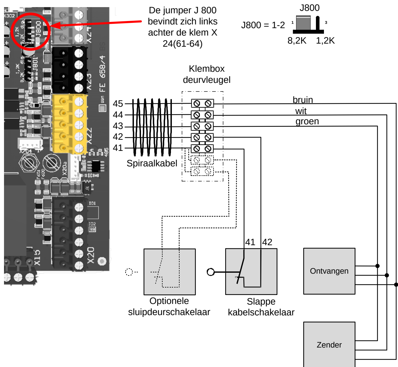
Afbeelding 19: Aansluiting optische veiligheidsstrip
