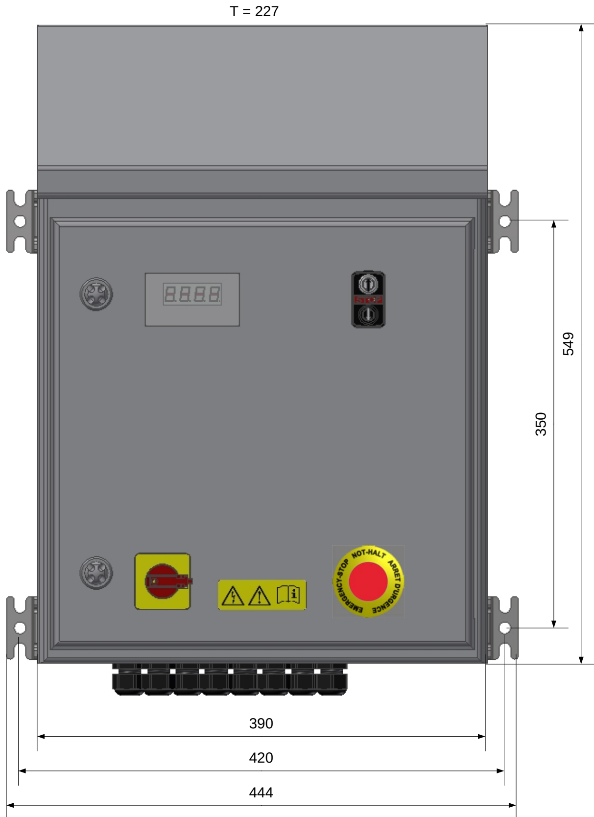
Afbeelding 15: Hygiënische behuizing (Typ: HYG)
