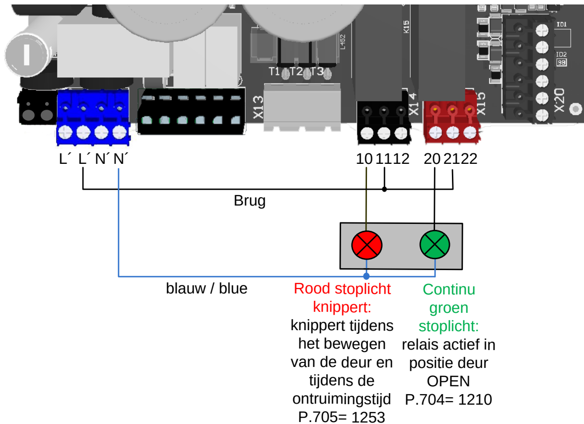
Afbeelding 32: Aansluiting van het stoplicht
