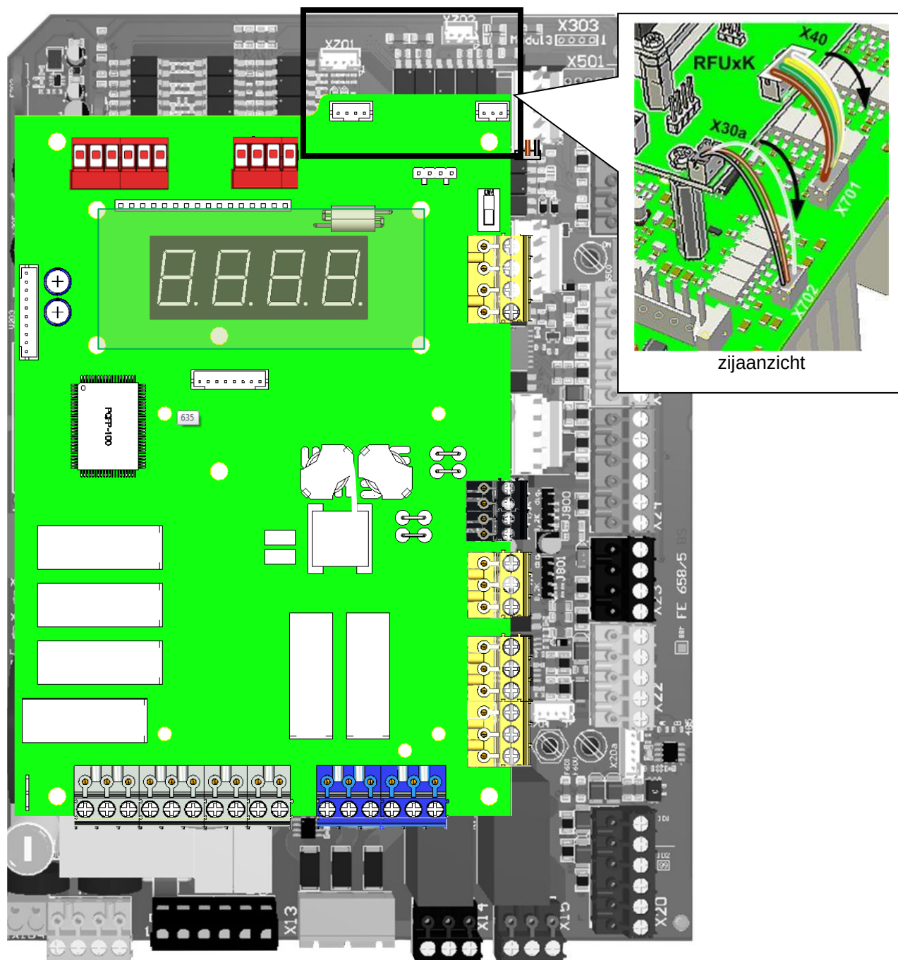
Afbeelding 39: TST RFUxK uitbreidingskaart aansluiten
