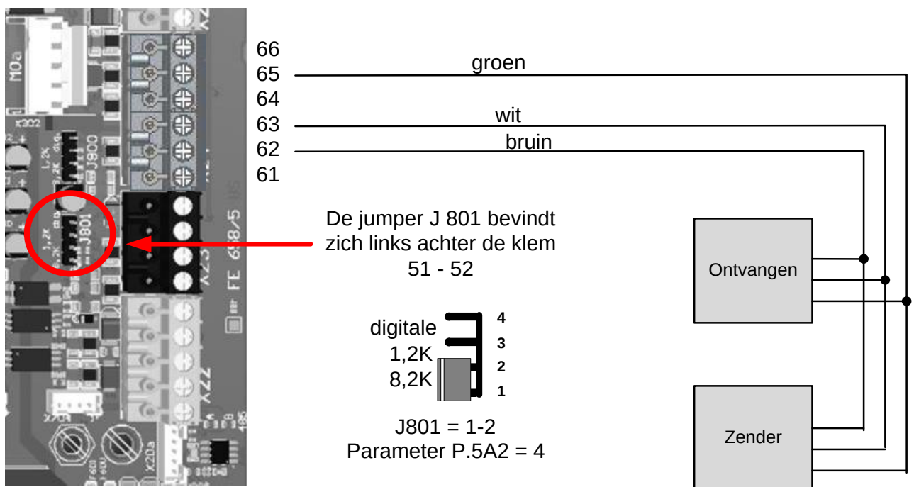
Afbeelding 21: Aansluiting optische veiligheidsstrip
