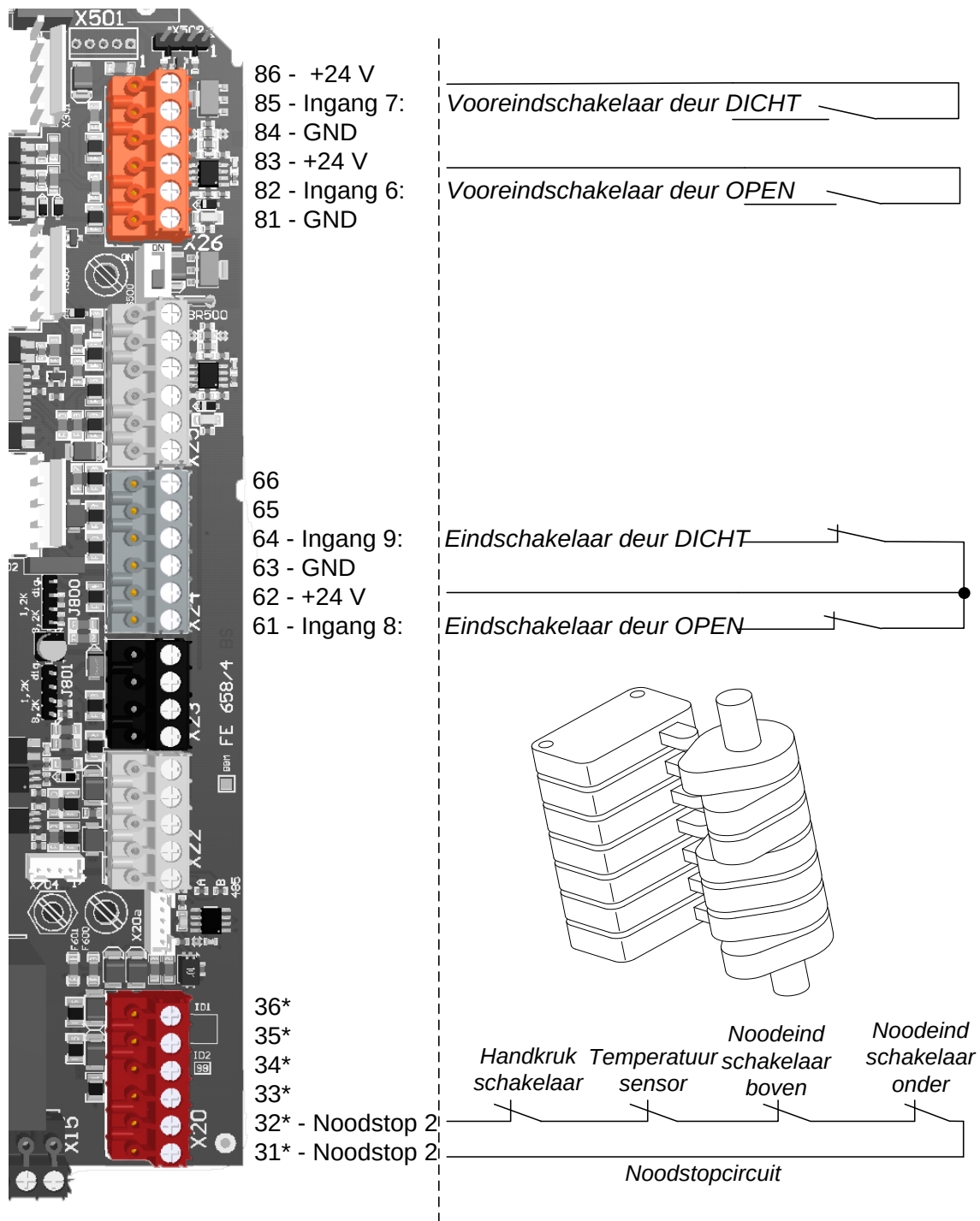
Abbeelding 29: Aansluiting nokkeneindschakelaar
