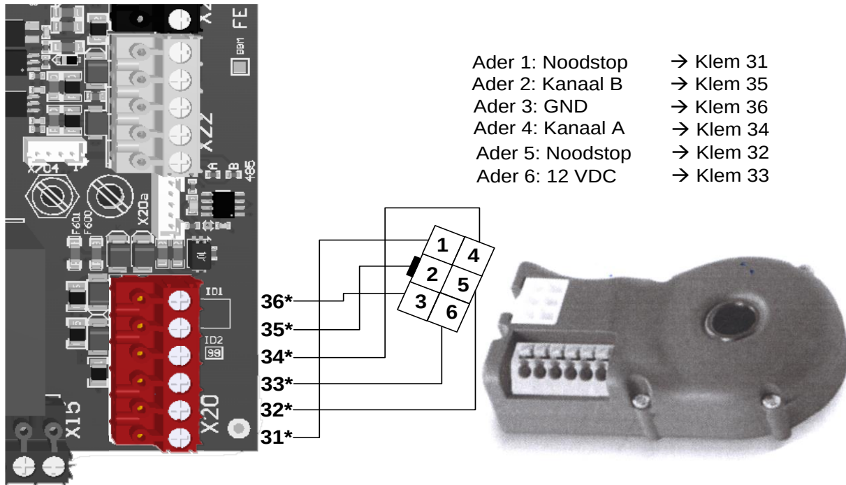
Afbeelding 28: Aansluiting absolute encoder DES
