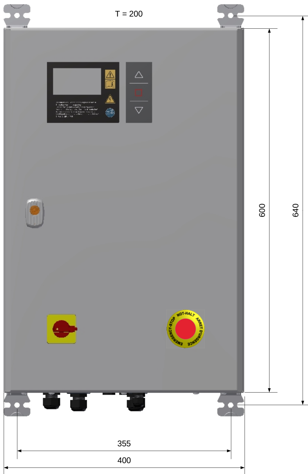
Afbeelding 12: Behuizing 400 x 600
