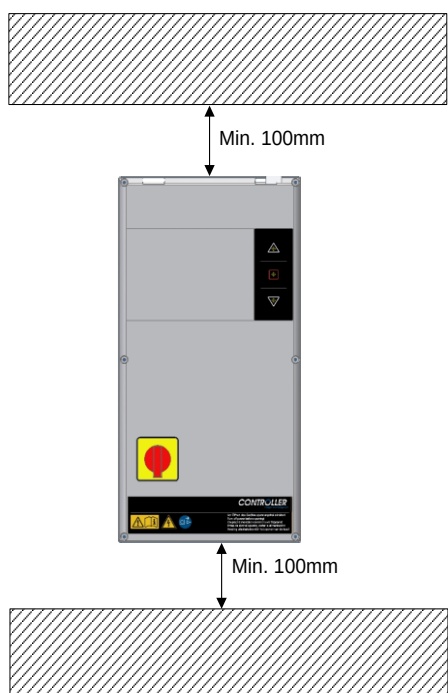
Afbeelding 9: Montage grote behuizing
