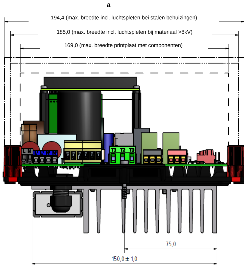
Afbeelding 2: Van onderen gezien
