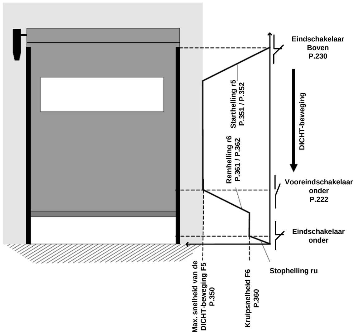
Afbeelding 48: DICHT-beweging met frequentie-omzetter
