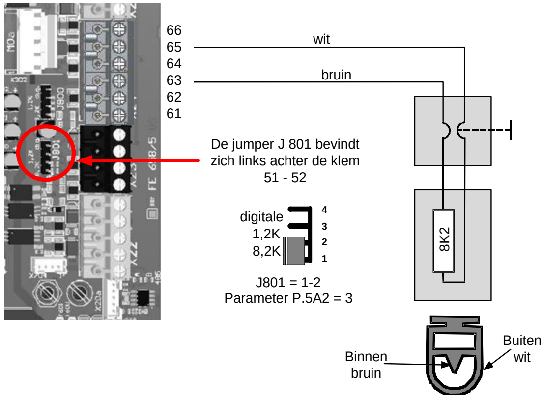
Afbeelding 22: Aansluiting van een weerstands- veiligheidsstrip
