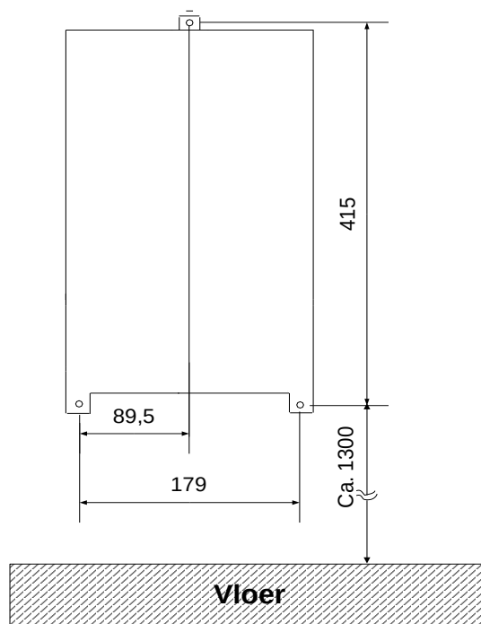
Afbeelding 10: Boorschema van grote behuizing
