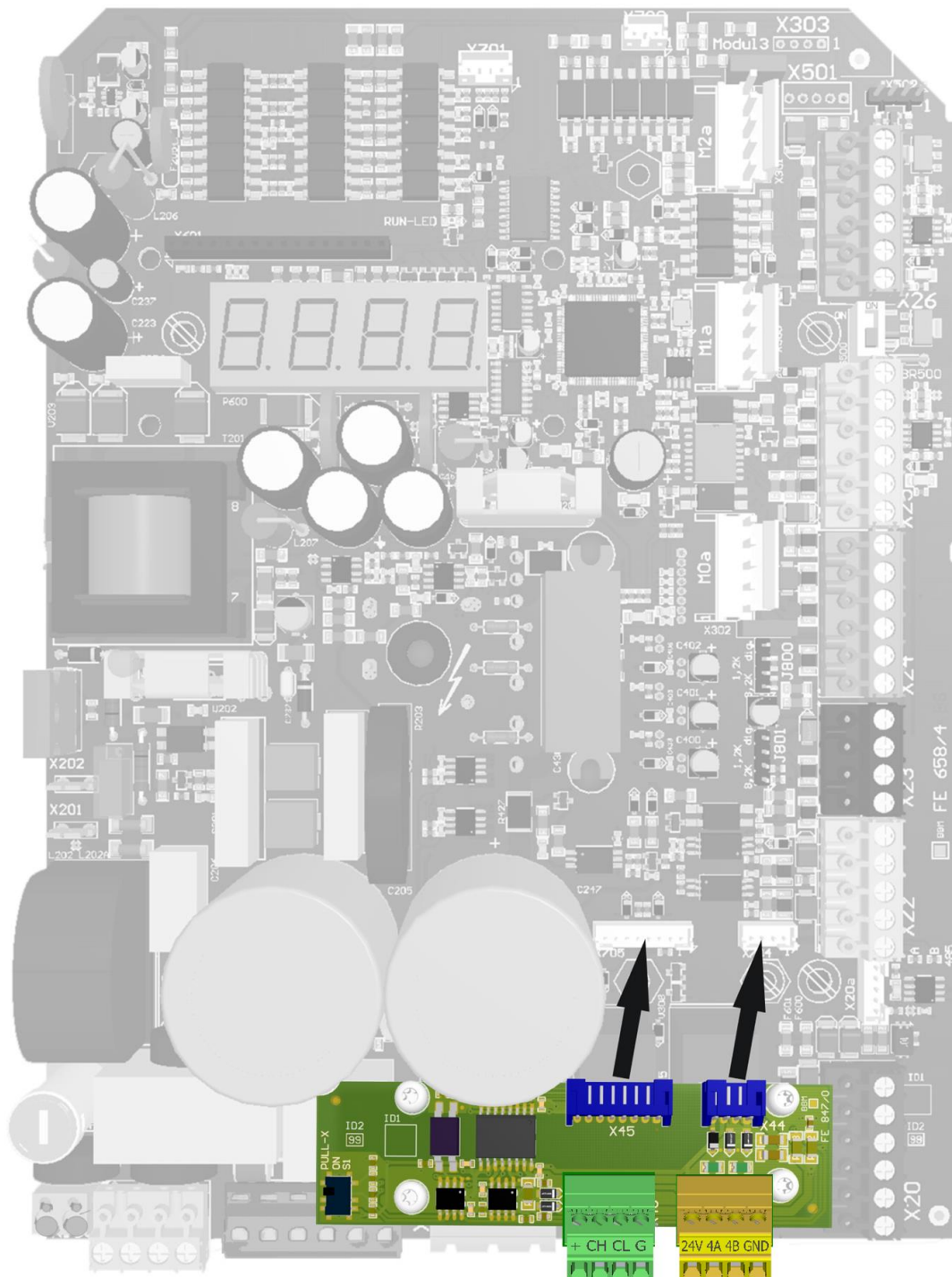
Afbeelding 40: Interfacekaart RFuXFCOM
