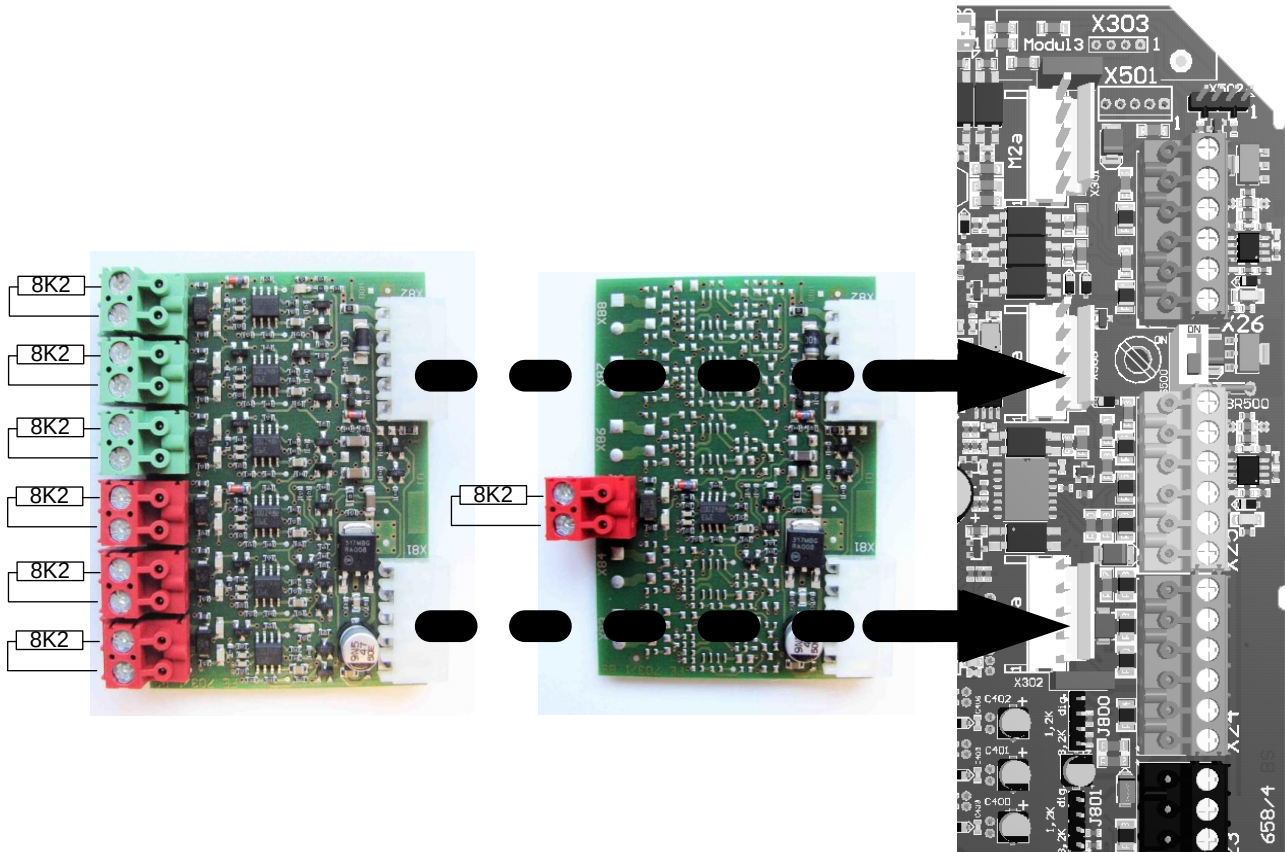
Afbeelding 38: Veiligheidsstripanalyse
