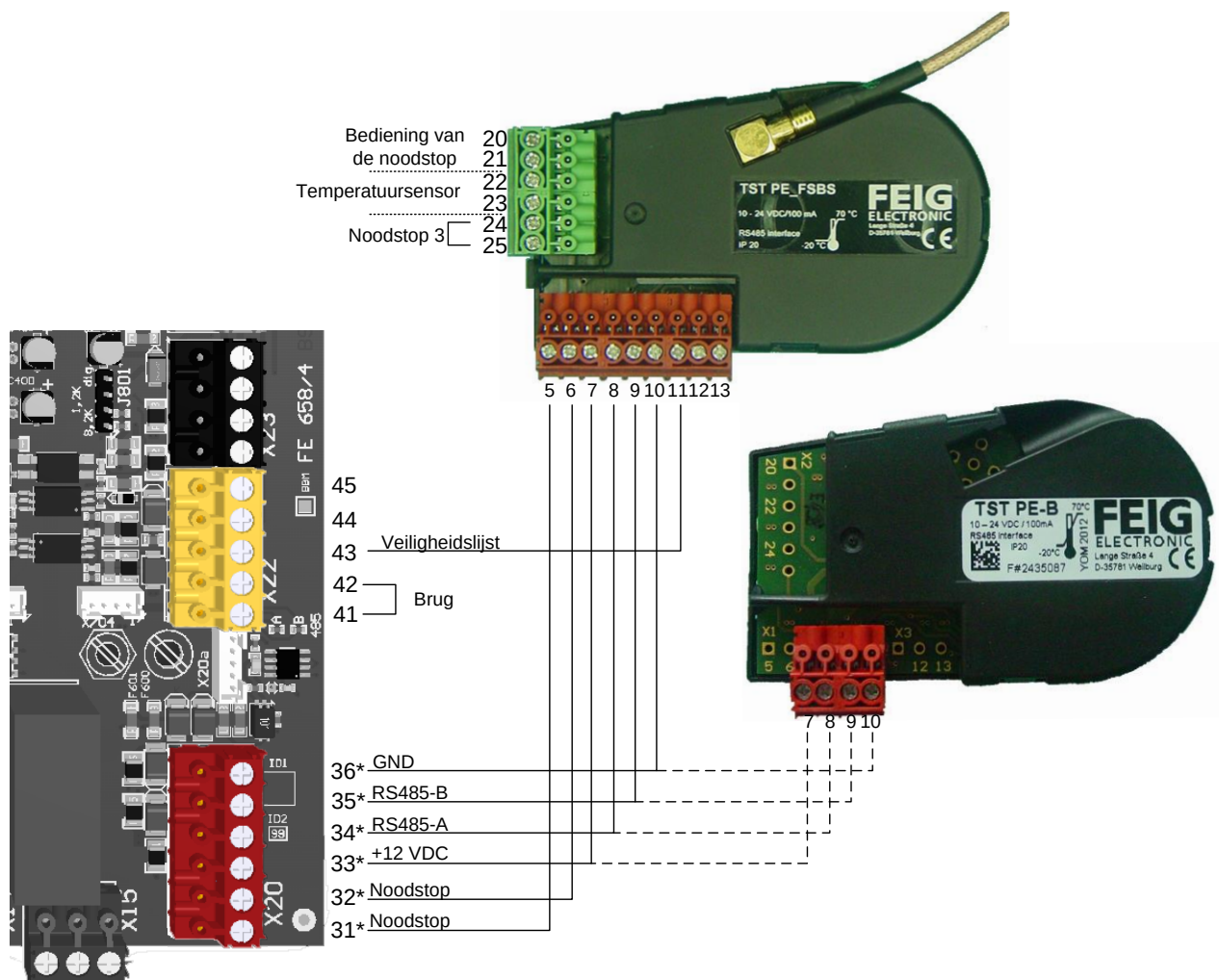
Afbeelding 26: Absolute encoder TST PE / TST PE FSB
