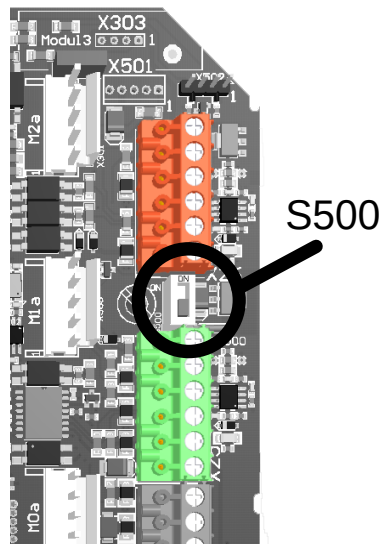
Afbeelding 44: Positie DIP- schakelaar
