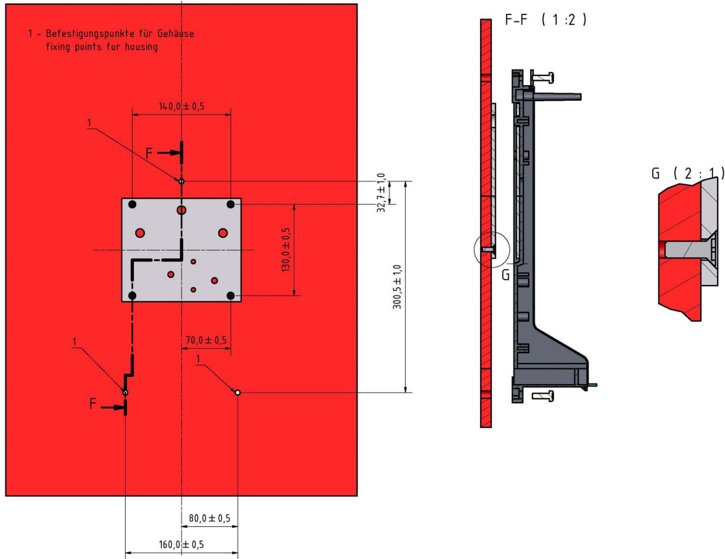
Afbeelding 8: Boorschema voor extra koellichaam en besturing
