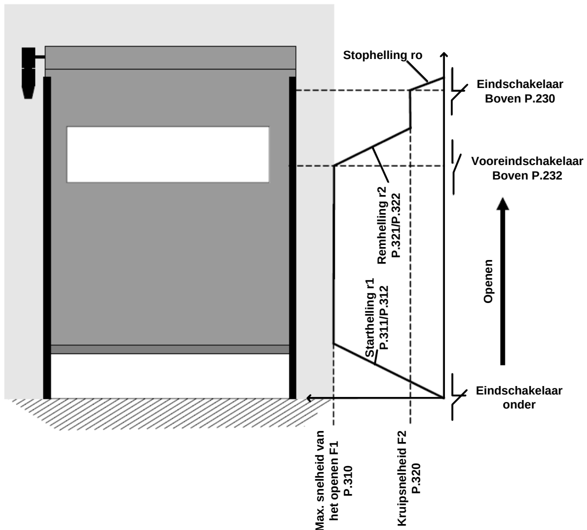
Afbeelding 47: Openen met frequentie-omzetter
