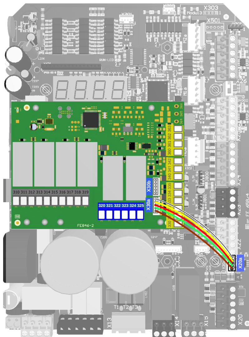
Afbeelding 42: Aansluitingsvoorbeeld met TST RFUxIO-E
