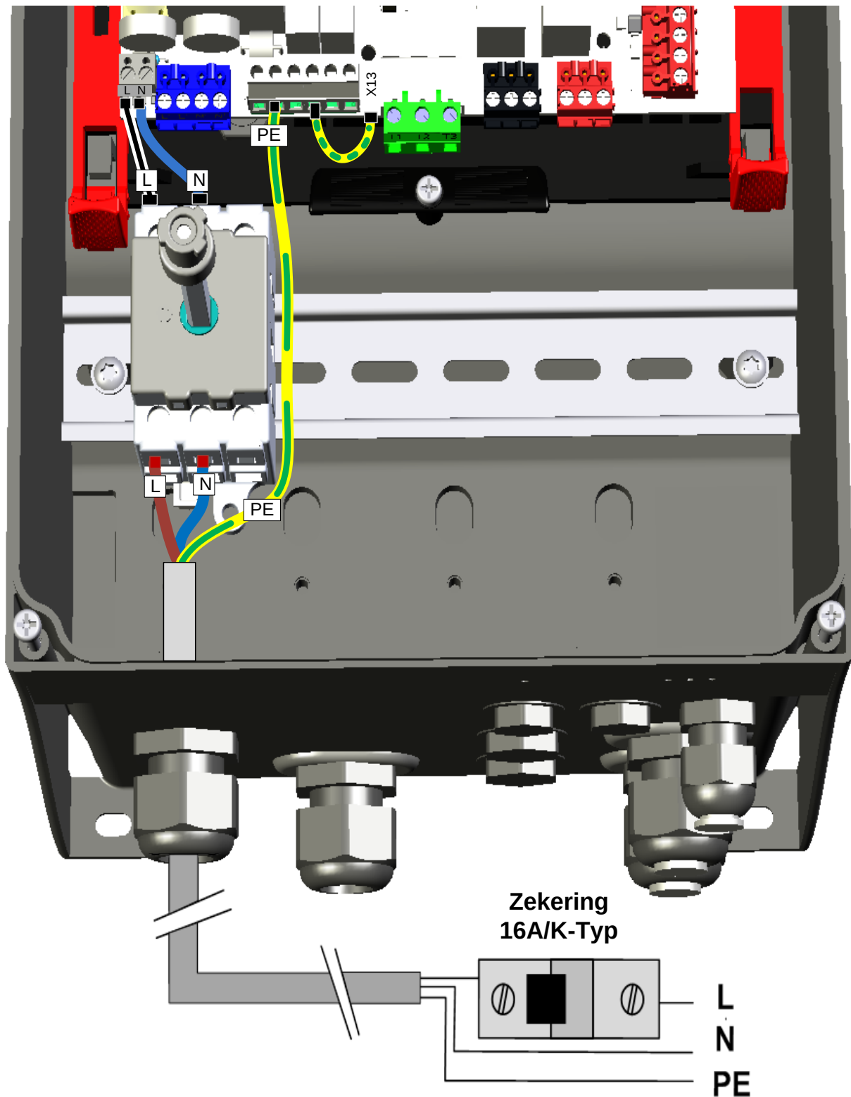
Afbeelding 17: Aansluiten van de netsnoer
