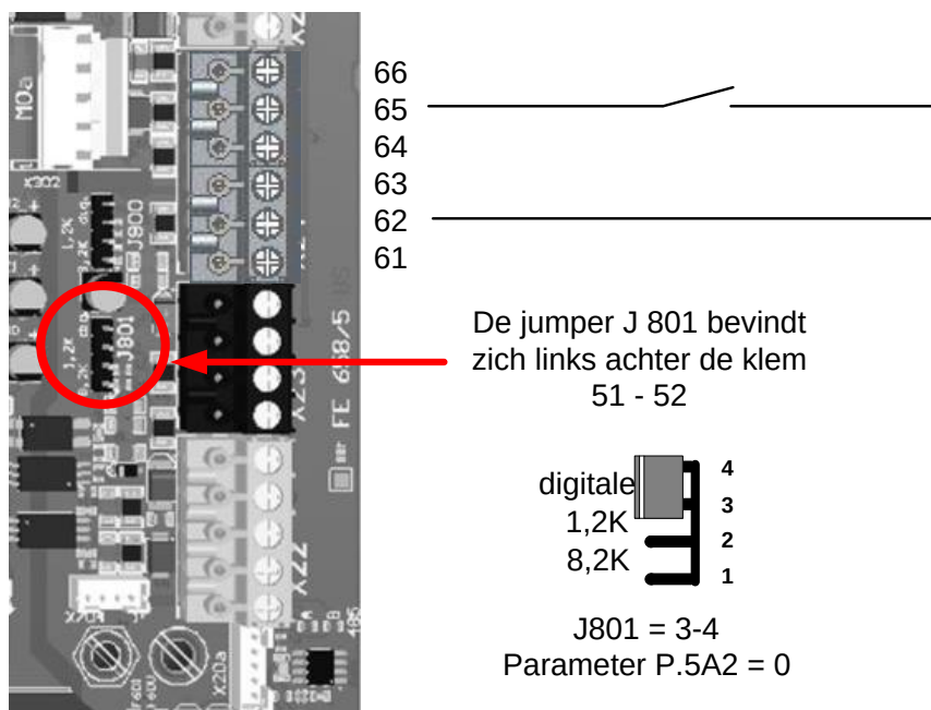
Afbeelding 23: Aansluiting van een weerstands- veiligheidsstrip
