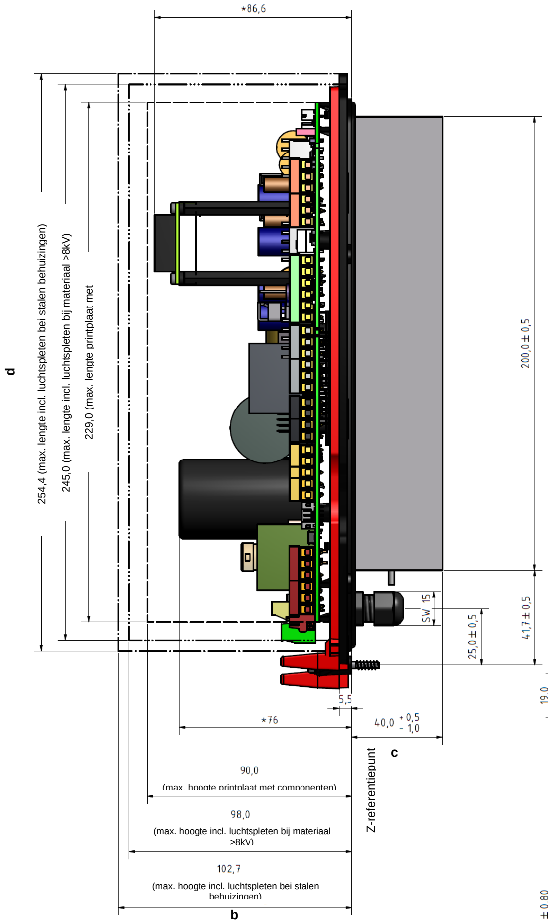
Afbeelding 3: Zijaanzicht
