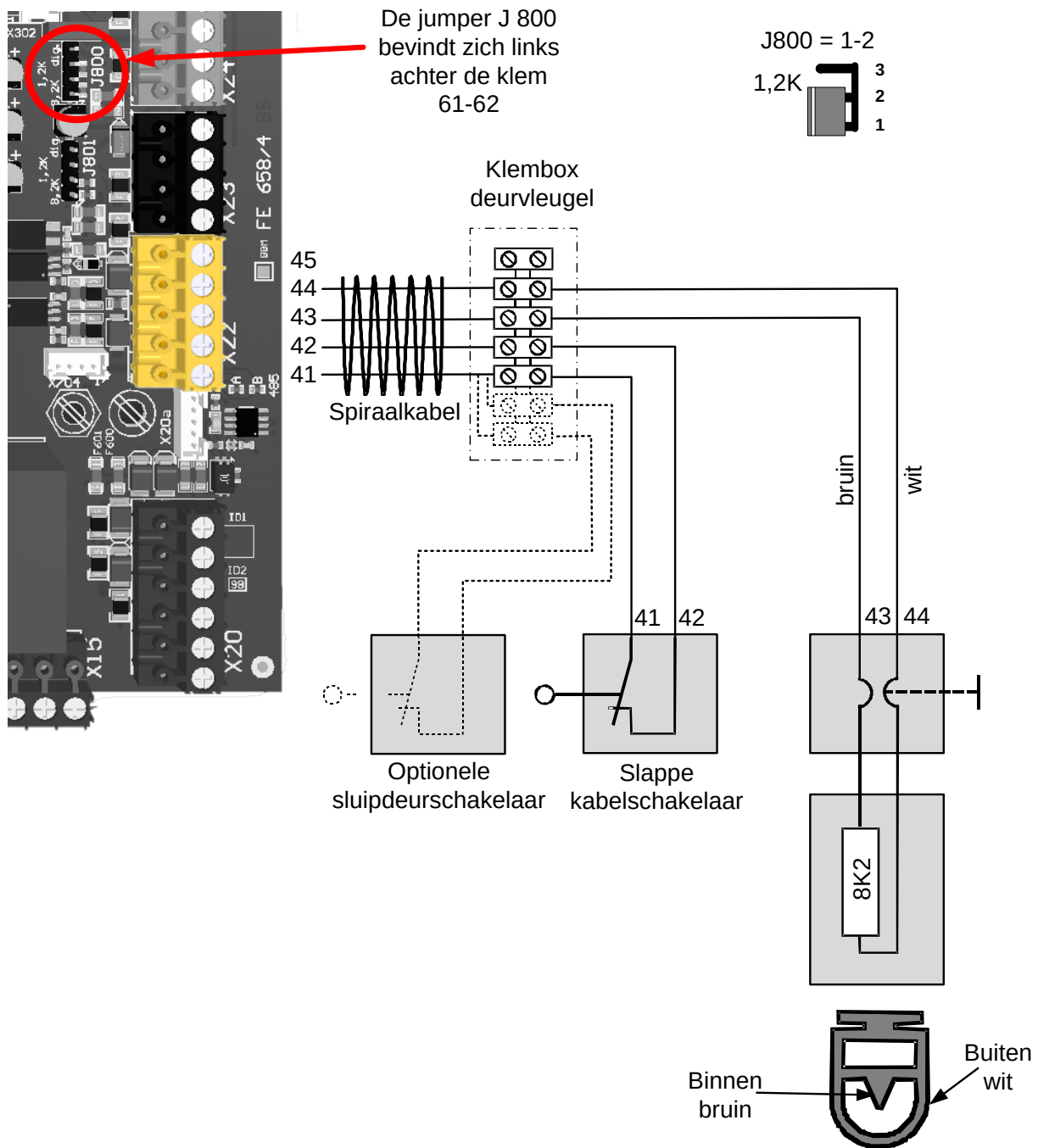
Afbeelding 20: Aansluiting van een weerstands- veiligheidsstrip
