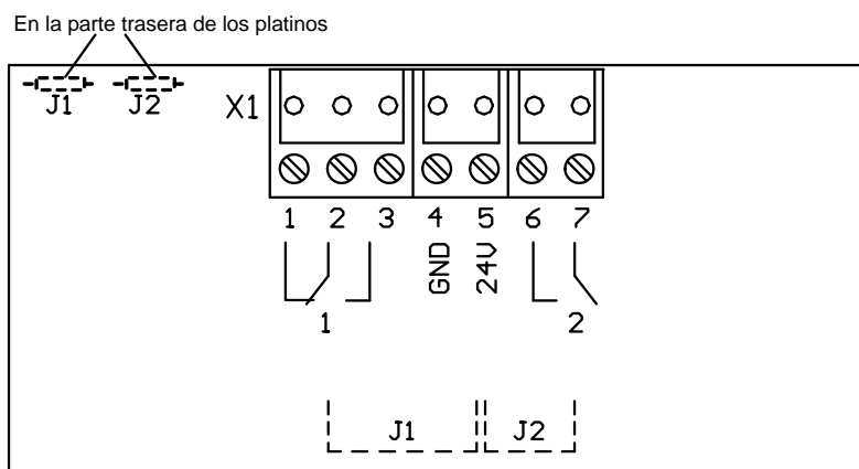
Ilustración 5: Bornes de conexión en platinos parte trasera
