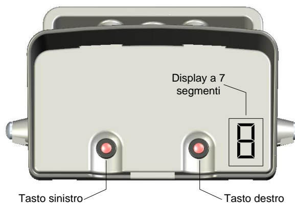
Figura 7: comando mediante tasti
