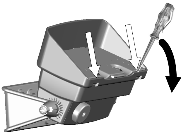
Figura 3: Apertura dell'involucro
