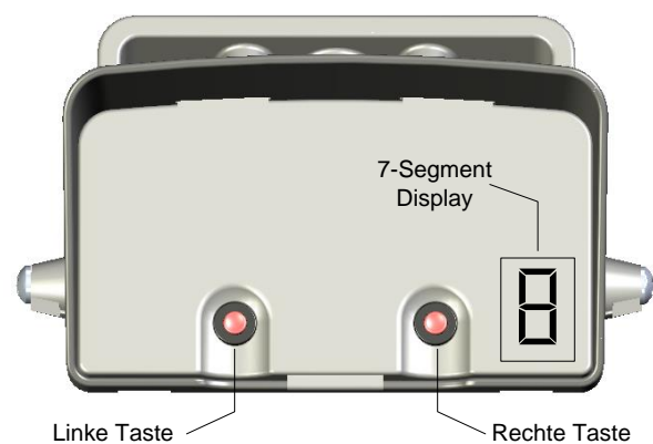
Abbildung 7: Bedienung über Taster
