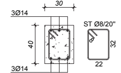
SECTION POUTRE DE LIAISON Échelle 1:20
