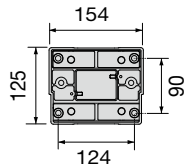
BEVESTIGINGSPLAAT ONDERDEELCODE 999533
