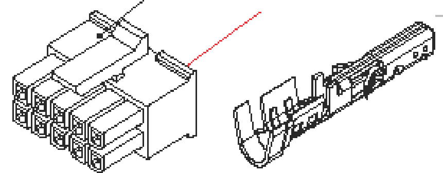
Kabelzuleitung
