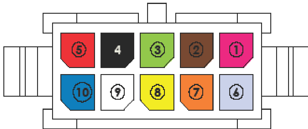
Vorderansicht
