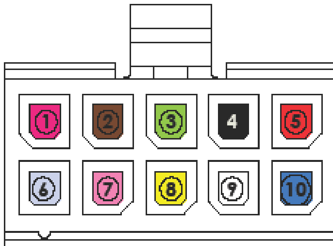
Vorderansicht
