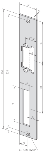
ProFix 1 vlakke sluitplaat, RVS, voor de ProFix 1-modellen (universeel) X-maat 14,5 mm
