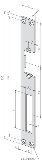
HZ vlakke sluitplaat, RVS, voor de modellen 143
