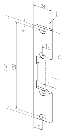
KL Profix-2 vlakke sluitplaat RVS, voor de Profix-2 modellen
